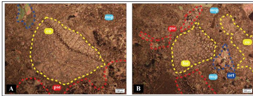
Gambar 18 Pengamatan Sayatan XPL Batugamping Grainstone (A) Dengan Bioklas Melimpah Seperti Lepidocyclus (B) Fosil Hadir Dalam Bentuk Pecahan-Pecahan Dengan Tanda Garis Warna Kuning yang Beberapa Telah Tergantikan Menjadi Sparit Semu Dengan Tanda Garis Merah.
