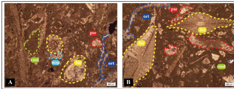
Gambar 7 (A) Wackestone Dengan Mikrit Melimpah dan Butiran Bioklas Hadir Seperti Lepidocyclus (For), (B) Fosil Lepidocyclus (Nephrolepidina) Parva Oppenoorth (Lo) Dengan Tanda Garis Warna Kuning.
