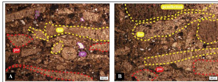
Gambar 9 Pengamatan Sayatan XPL Batugamping Floatstone (A) Dengan Bioklas Melimpah Dan (B) Fosil Hadir Dalam Bentuk Utuh Dengan Tanda Garis Warna yang Telah Termikritkan Karena Proses Galian Organisme.
