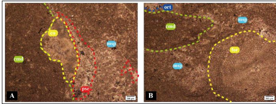
Gambar 16 Pengamatan Sayatan XPL Batugamping Floatstone (A) Bioklas Yang Hadir Berupa Coral In Situ Dan (B) Fosil Yang Hadir Dalam Bentuk Utuh Dengan Tanda Garis Warna Kuning Merupakan Lepidocyclina (For) Yang Berada Dalam Matriks.
