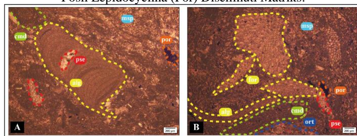
Gambar 11 Pengamatan Sayatan XPL Batugamping Wackestone (A) Dengan Bioklas Berupa Alga Merah (Alg) Diselimuti Matriks Berupa Lumpur Karbonat dan Mikrit Telah Mengalami Rekrystalisasi atau Mikrosparit (Msp) dan (B) Fosil Lepidocyclina (For) dan Alga Merah.
