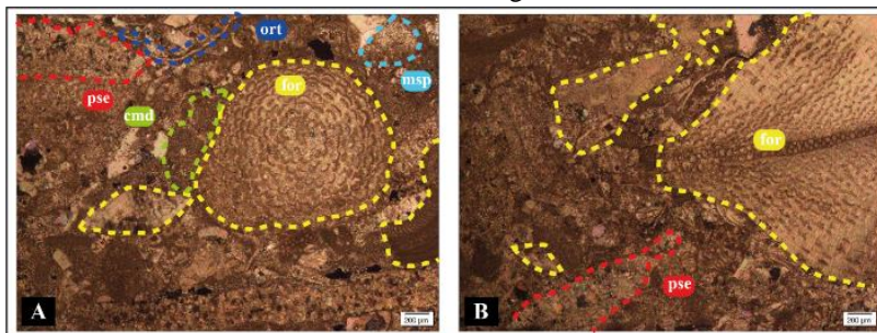
Gambar 6 (A) Floatstone Bioklastika Dengan Beberapa Butiran Skeletal Seperti Lepidocyclina (For), (B) Fossil Lepidocyclina Yang Memiliki Ukuran Rata-Rata > 2 mm.
