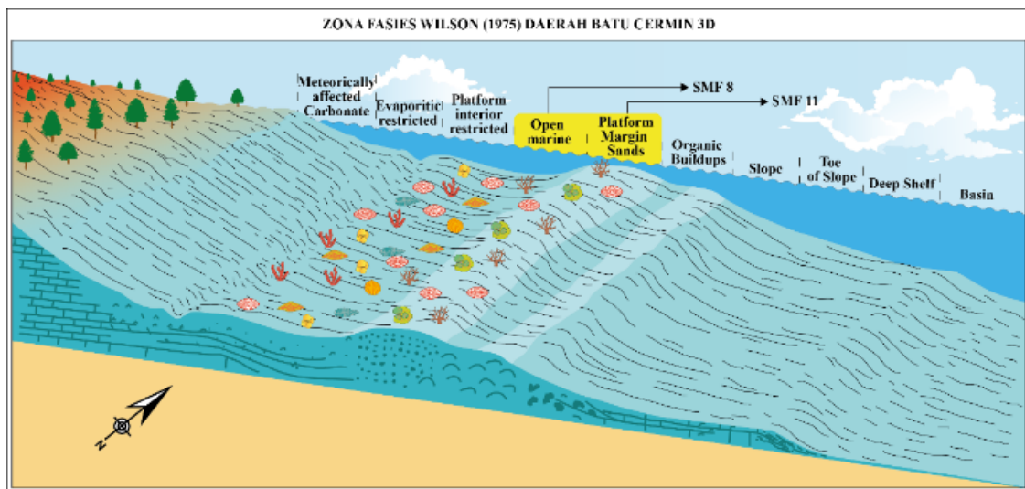
Gambar 22 Model Pengendapan Batugamping Daerah Batu Cermin Formasi Bebuluh Mengacu Pada Standard Microfacies Types Menurut Flügel (1982) Serta Sabuk Fasis Didasarkan Kepada Paparan Karbonat Terbatas Pada Daerah Tropis (FZ) yang Diusulkan Oleh Wilson (1975).
