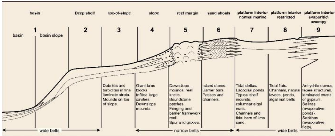
Gambar 3 Rimmed Platform (FZ) Oleh Wilson yang Dimodifikasi Pada Buku Carbonate Sedimentology and Sequence Stratigraphy (Schlager, 2005)
