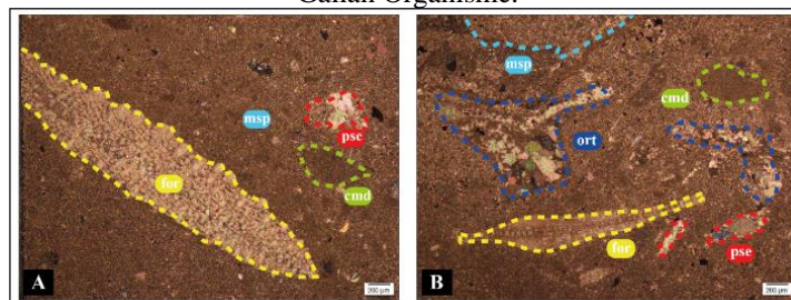
Gambar 10 Pengamatan Sayatan XPL Batugamping Wackestone (A) Kenampakan Fosil Miogypsina Kotoi (Hanzawa, 1931) Di Dalam Matriks Lumpur Karbonat (B) Fosil Hadir Dalam Bentuk Utuh Yaitu Fosil Lepidocyclina (For) Diselimuti Matriks.
