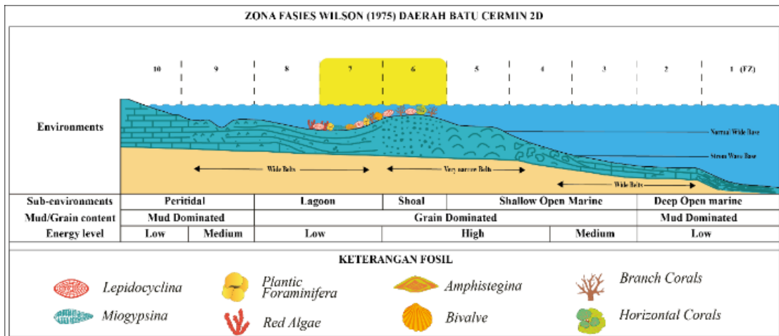
Gambar 21 Model Pengendapan Batugamping Daerah Batu Cermin Formasi Bebuluh Mengacu Pada Standard Microfacies Types Dikemukakan Flügel (1982) Dan Sabuk Fasies Didasarkan Kepada Paparan Karbonat Terbatas Di Daerah Tropis (FZ) Diusulkan Oleh Wilson (1975) Dalam 2D.
