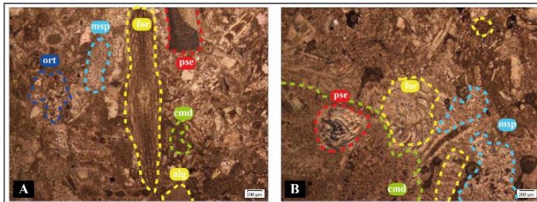
Gambar 4 (A) Wackestone Bioklastika Dengan Butiran Skeletal Seperti Lepidocyclina (For), (B) Terdapat Fosil Amphistegina (For) Yang Telah Tergantikan Menjadi Sparit Semu Atau Pseudosparit
